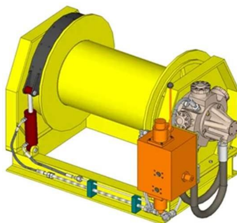
Tời kéo/nâng thủy lực
